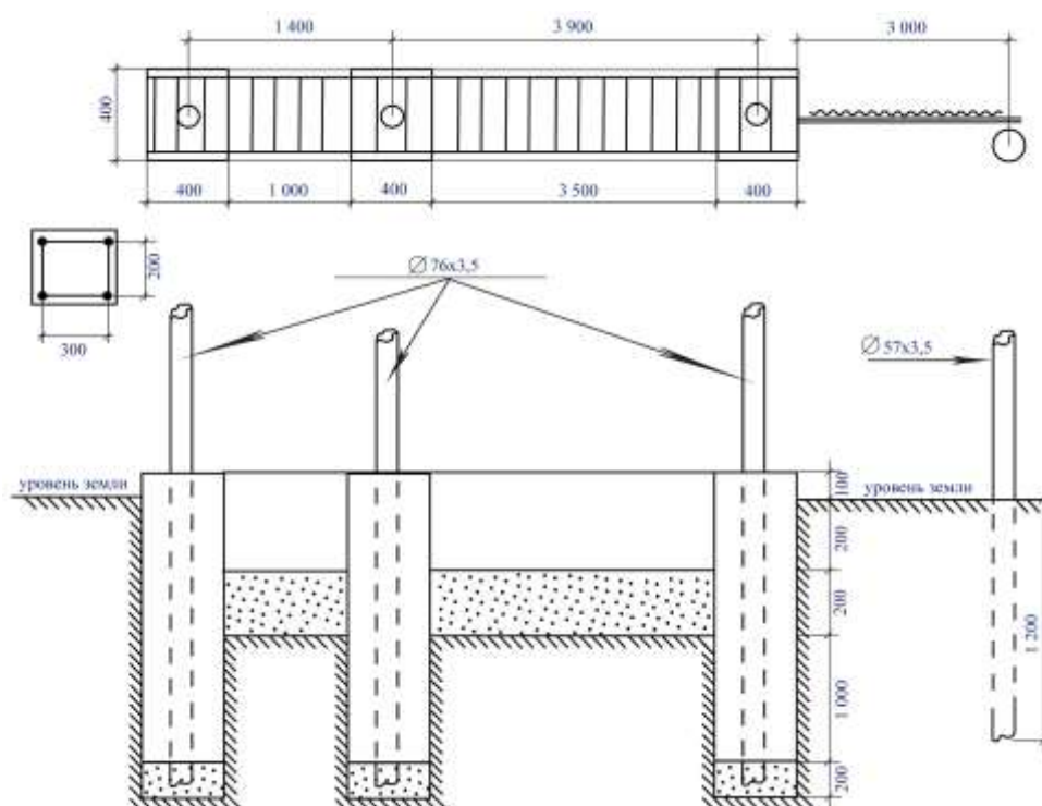
Схема забора. Лист 1.
